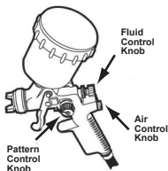
(Dwg. TP2268)
